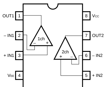
BA4560 / BA4560F
